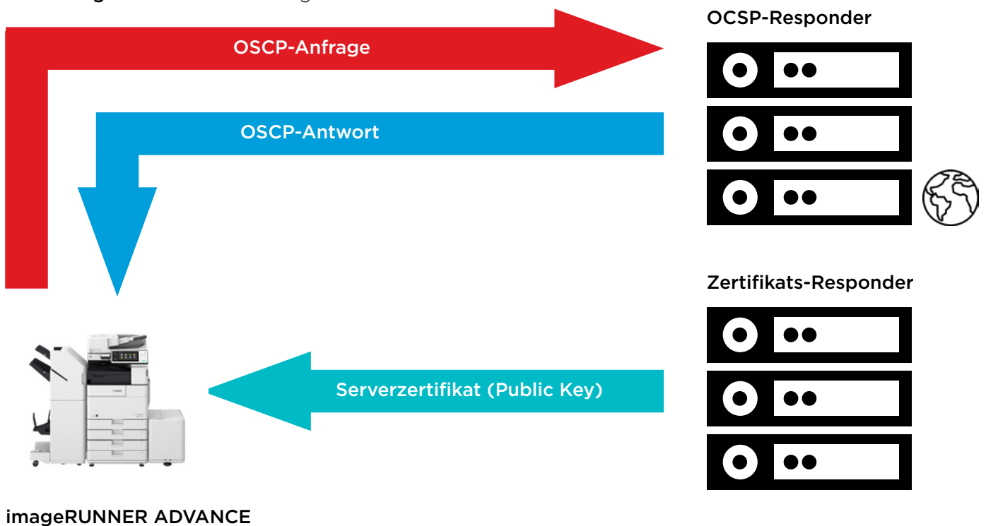
Abbildung 6 OCSP-Handshaking-Prozess
